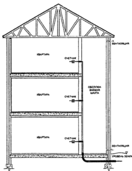
Рисунок Г.2. Газопровод в вентилируемой шахте
